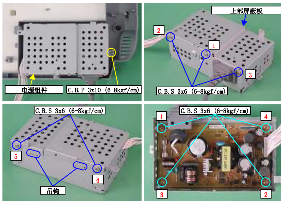
图 2-37. 电源组件拆卸
