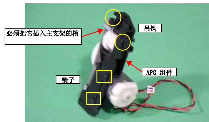
图 2-19. APG 组件安装
