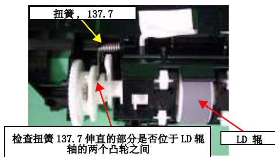
图 2-16. “扭簧 137.7 的位置”
