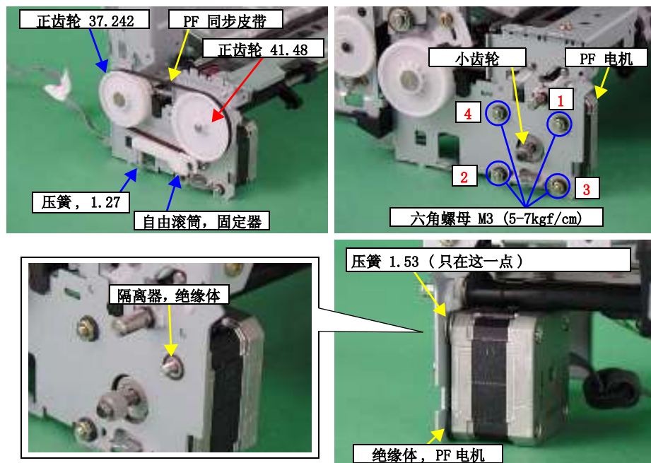
图 2-49. PF 电机拆卸
