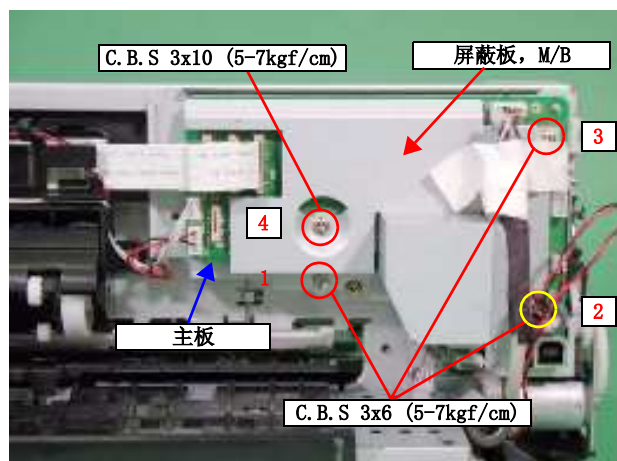
图 2-12. 主板拆卸
