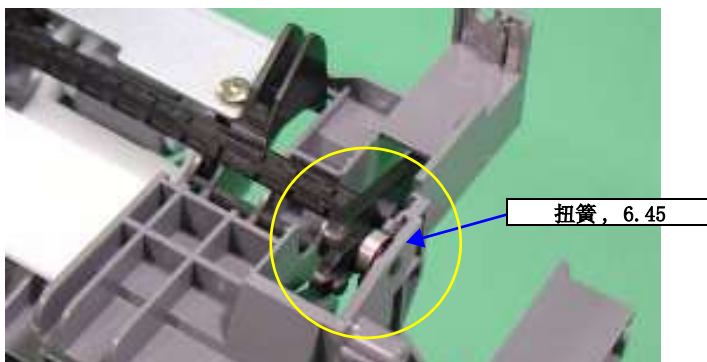
图 2-7. 拆卸“扭簧，6.45”
