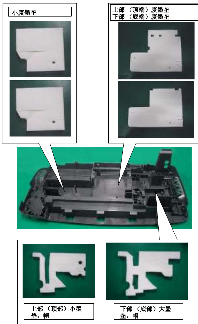
图 2-33. 废墨垫安装 (1)
